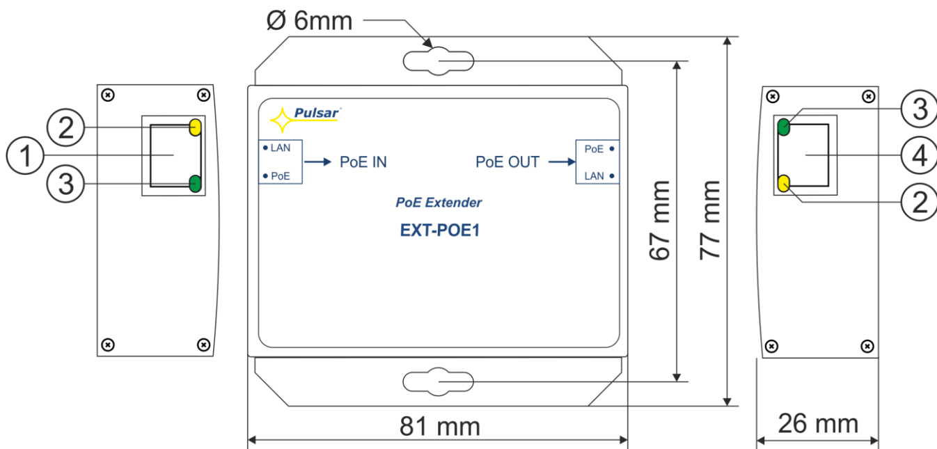
Rys. 2. Widok extender'a.
