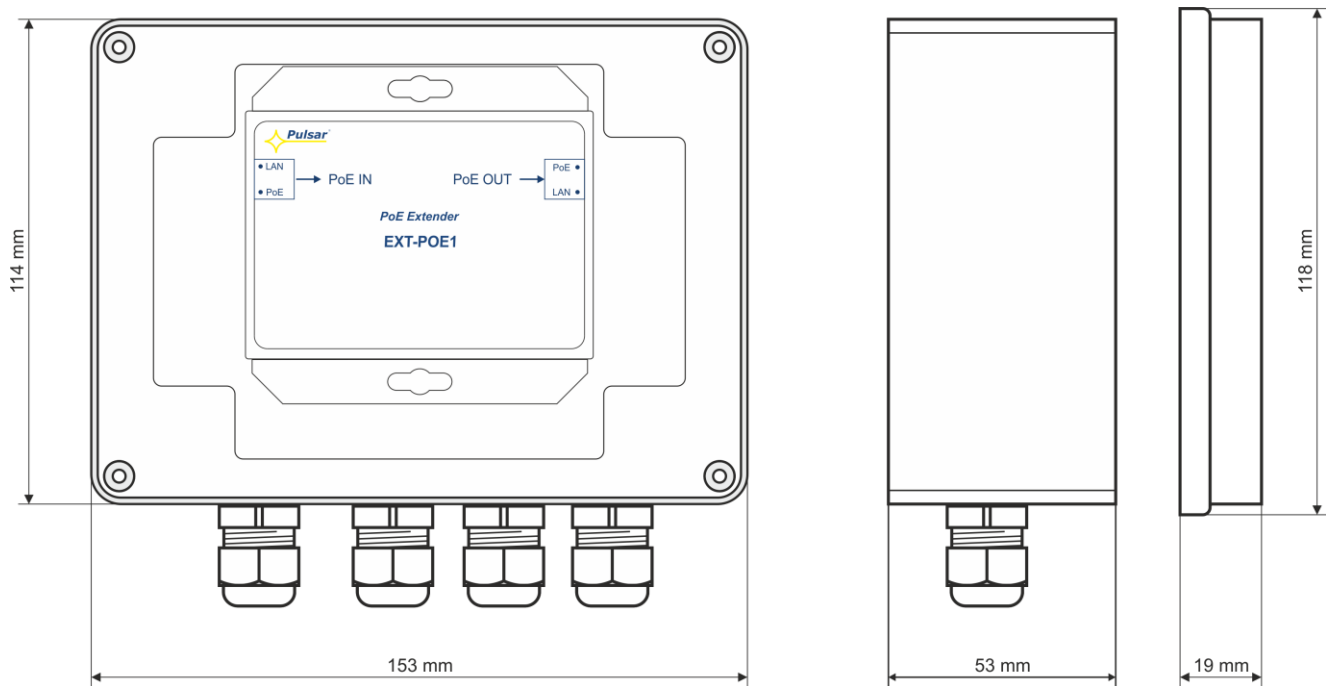
Rys. 1. Widok obudowy.
