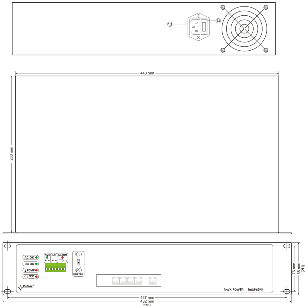
Rys.3. Widok zasilacza.
