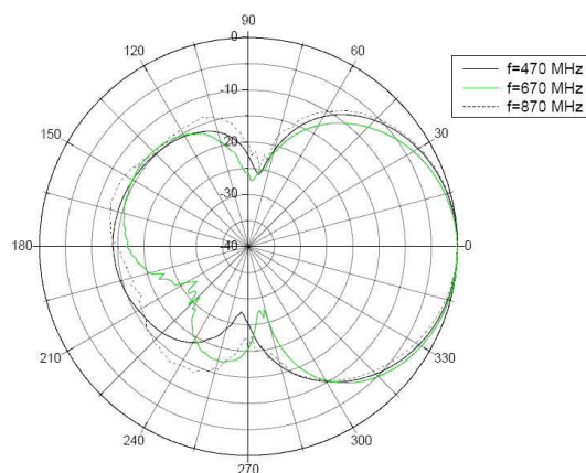
Charakterystyki promieniowania anteny w płaszczyźnie poziomej (Horizontal).
