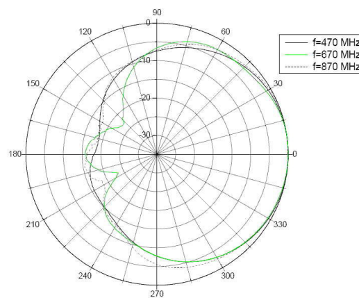
Charakterystyki promieniowania anteny w płaszczyźnie pionowej (Vertical).
